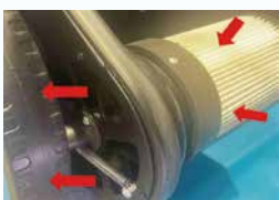
バキューム機能搭載。 ウォッシュアップフィルターと 換気ファン内蔵で本機内部が負圧の 状態を維持しダストの吹き出しを 大幅軽減。
